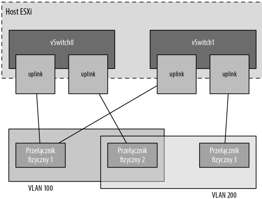
RYSUNEK 5.30. Wszystkie fizyczne karty sieciowe w grupie muszą przenosić te same VLAN-y
